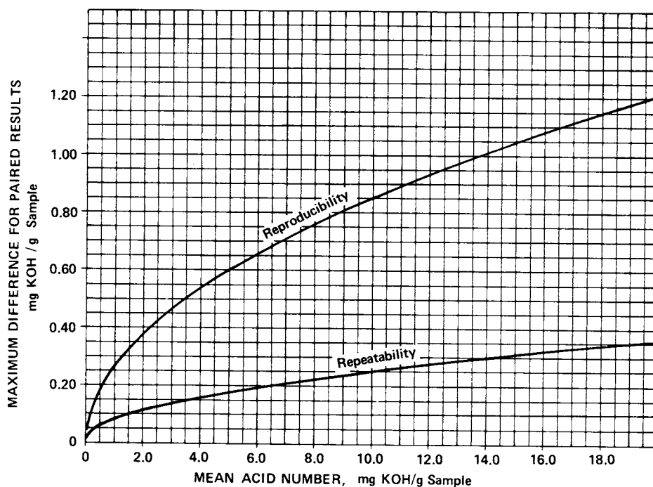
FIG. 2 Precision Curves
