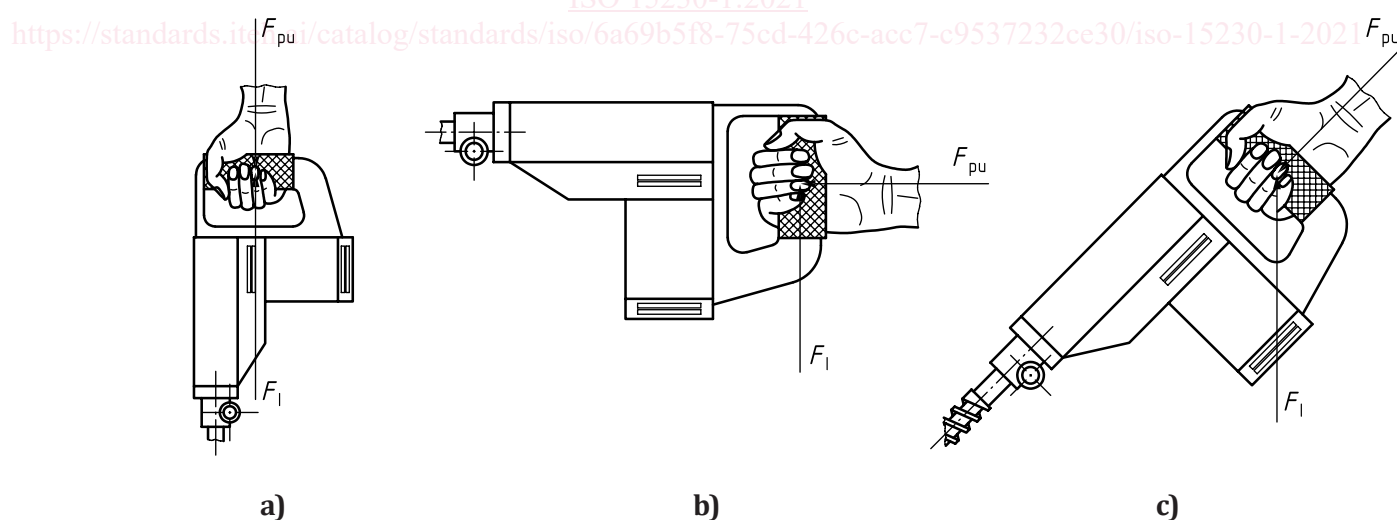
Figure 4 — Exemple de force de levage, F_l , avec indication d'une force de poussée, F_{pu}
