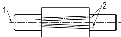
b) Écart de parallélisme
