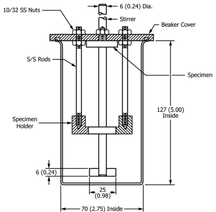
FIG. 1 Rusting Test Apparatus
