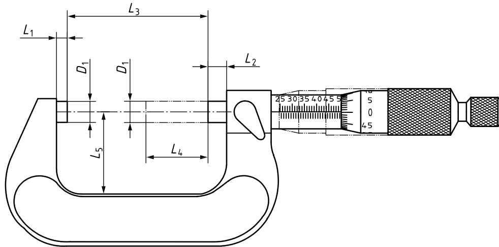
Figure 2 — Dimensions d'un micromètre d'extérieur
