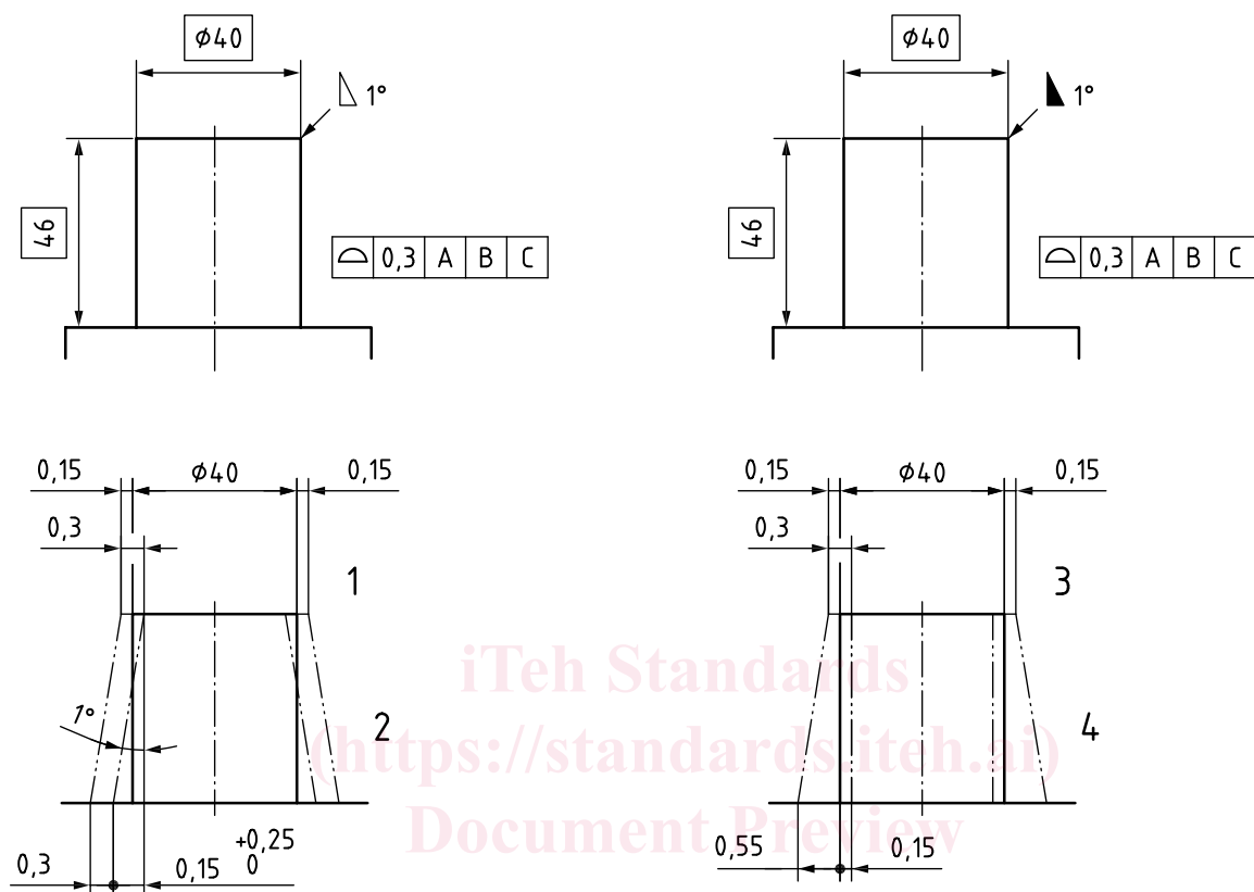
a) Angle de dépouille augmentant l'(les) élément(s) du modèle idéal
