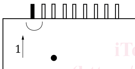
a) Activation du premier élément et front d'ondes se déplaçant dans l'objet contrôlé d) Front d'ondes juste avant son arrivée sur les éléments du réseau
