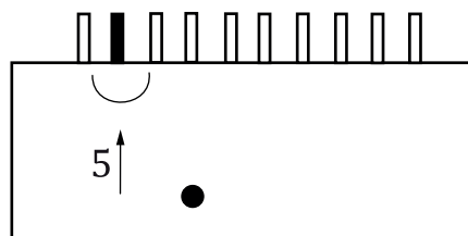
c) Écho(s) réfléchi(s) ou diffracté(s) de la discontinuité revenant en direction du réseau f) Processus se poursuivant par l'activation de l'élément 2 et se répétant jusqu'à ce que le dernier élément N du réseau ait été activé
