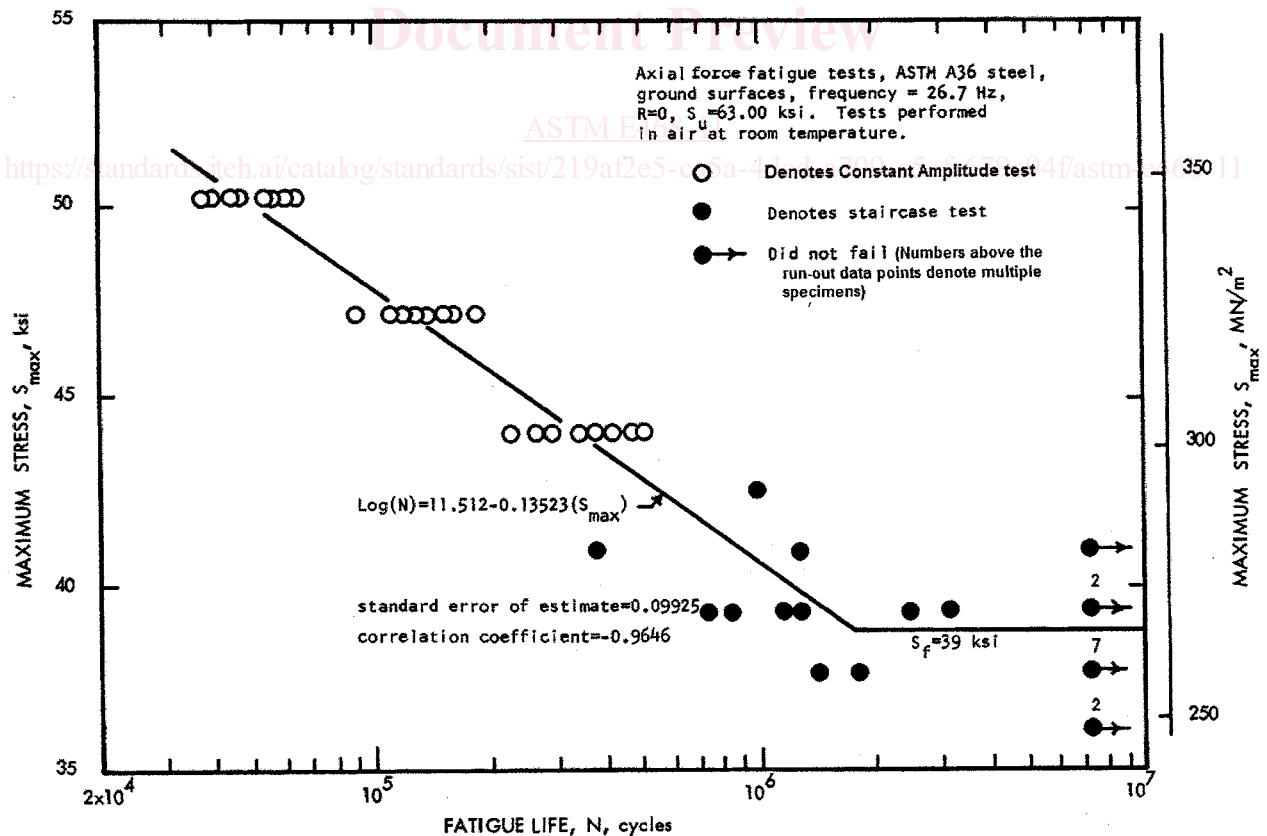
FIG. 1 S-N Diagram
