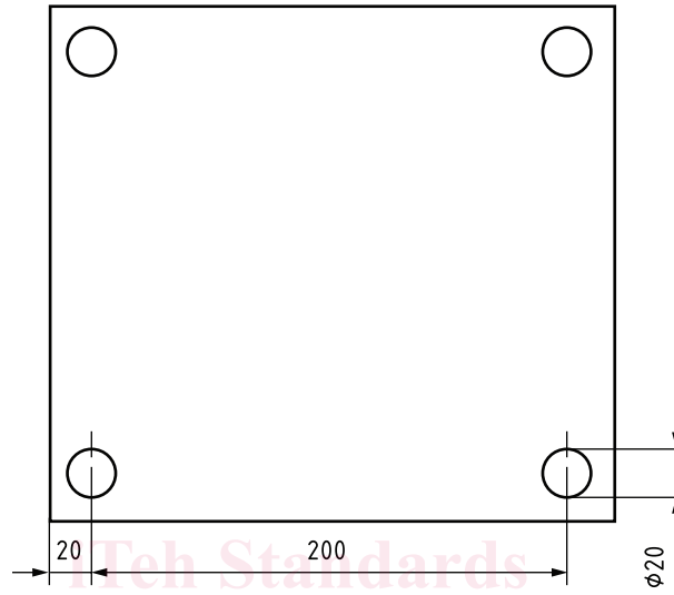
Figure 1 — Exemple de plaque d'acier rigide
