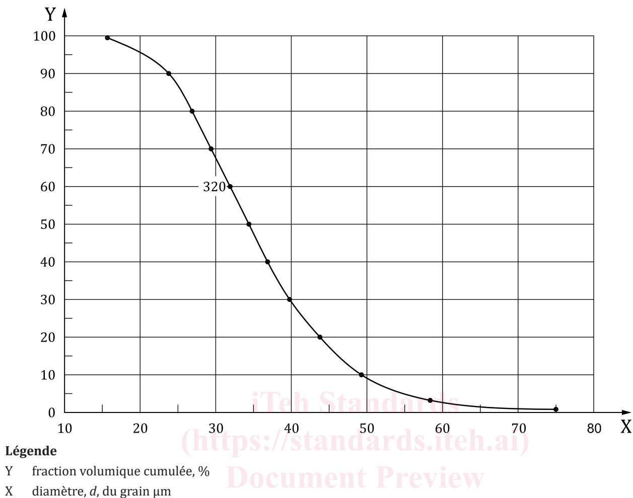
Figure 1 — Courbe de distribution granulométrique cumulée en volume du grain étalon 320
