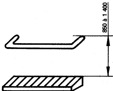
Figure 5 — Main courante au-dessus d'une passerelle
