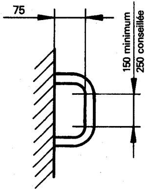
Figure 3 — Poignée
