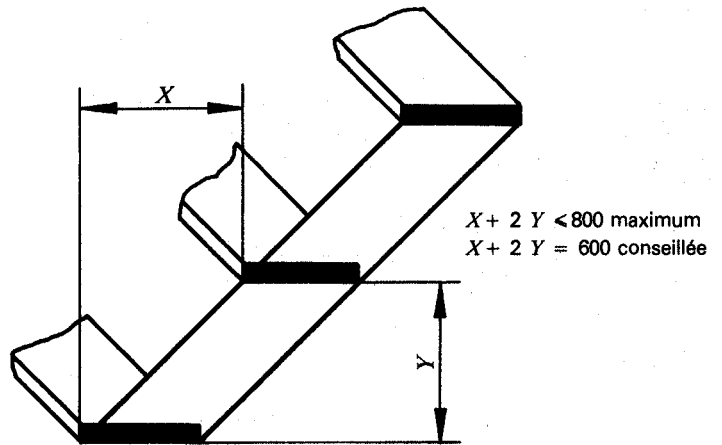
Figure 2 — Échelle
