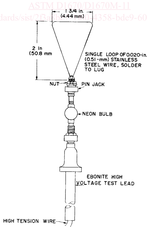
FIG. 1 Feeler
