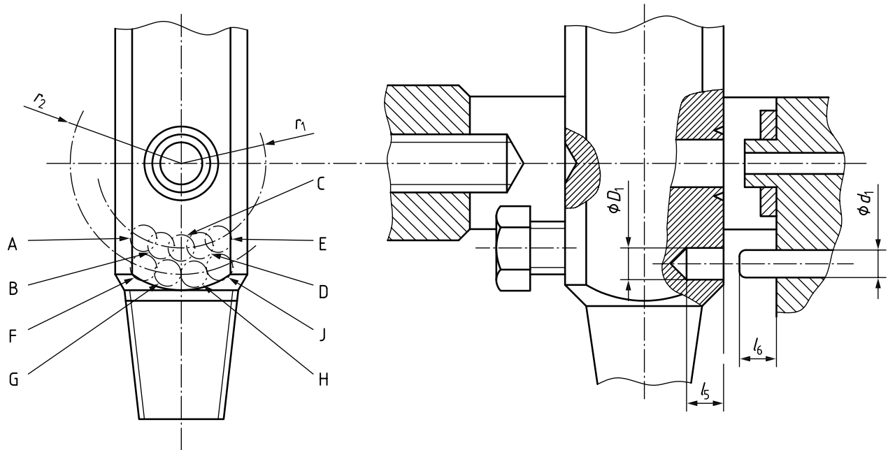
Figure 4 — Système de raccord de robinet du type étrier avec deux ergots de sécurité sur deux rangs
