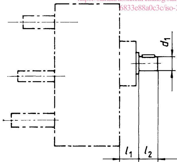
Figure 2 — Arbre d'entraînement
