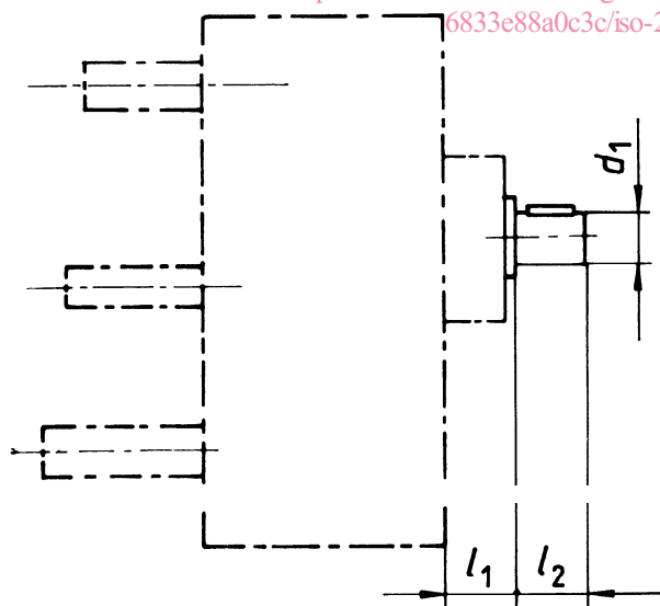
Figure 2 – Arbre d'entraînement
