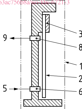
a) Éprouvette montée verticalement avec l'extrémité supérieure bridée (Méthode A)
