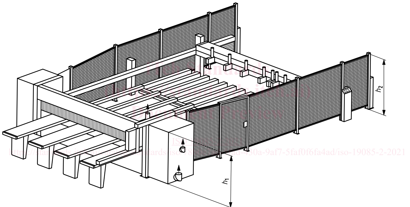
a) Exemple d'une machine à pousseur de panneau et chargement de panneaux par l'arrière par un dispositif de chargement mécanisé et avec barrière de maintien à distance et barrière lumineuse
