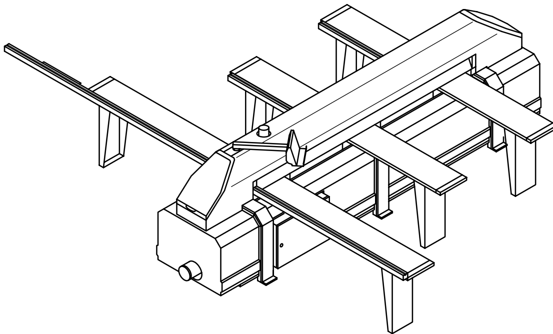
d) Exemple d'une machine sans pousseur de panneaux
