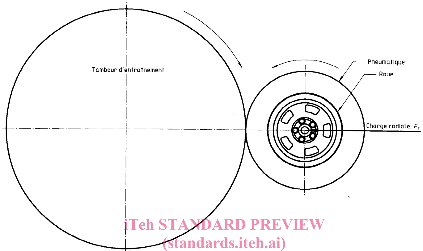
Figure 2 — Exemple de dispositif de montage pour l'essai de fatigue radiale
