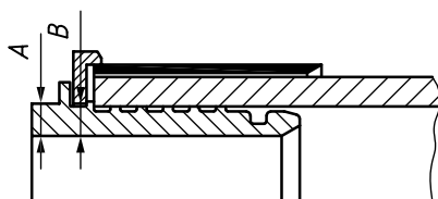
Figure B.2 — Exemple de raccord à sertissage axial (ou à glissement)
