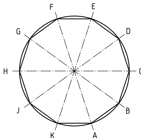
b) Vue en plan des stations horizontales
