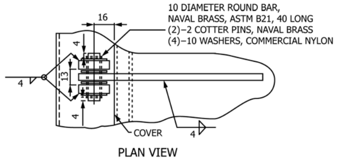
FIG. 2 Hinge
