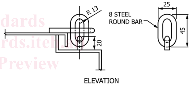
FIG. 2 Hinge
