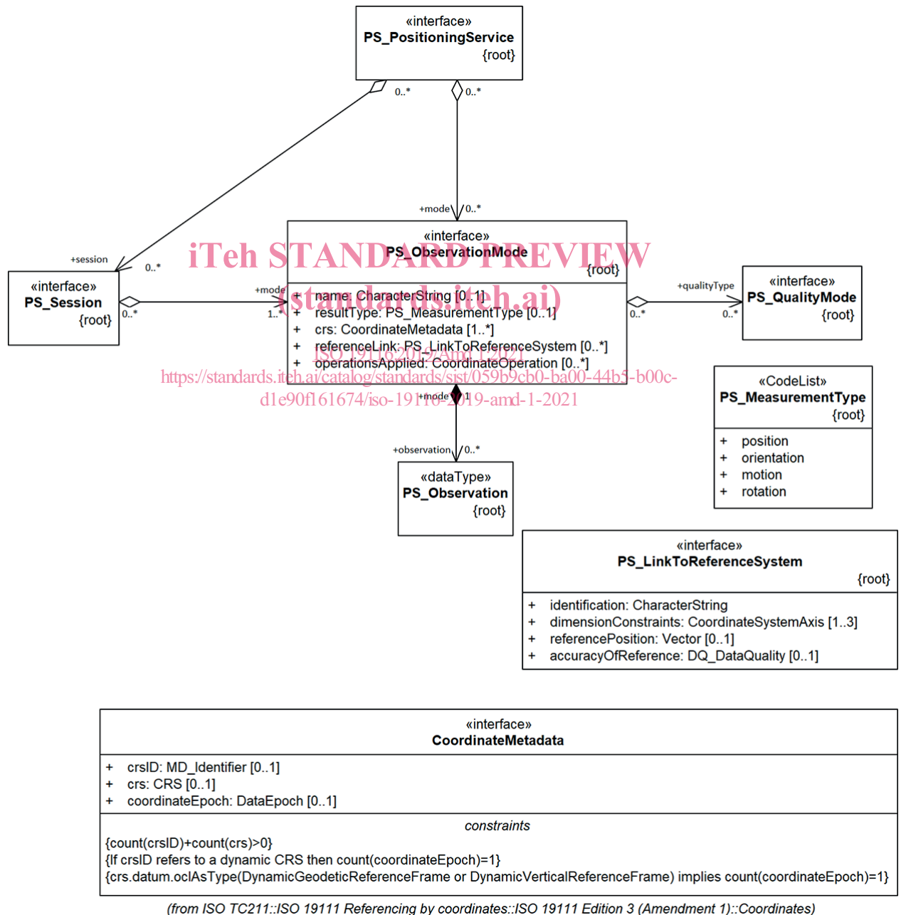
Figure 6 — Diagramme UML — Classe PS_ObservationMode et types de données associés
