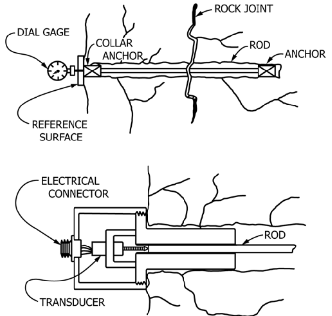
FIG. 1 Rod Extensometer
