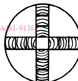
FIGURE 2 — Schéma du débit d'une planche de cœur d'une grume de diamètre égal ou inférieur à 180 mm admis dans l'échantillonnage systématique
