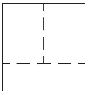
Figure 9 — Traits à un tiret se croisant comme une croix partielle
