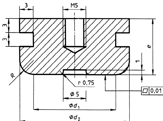
Figure 1 — Détails de l'éprouvette normalisée
