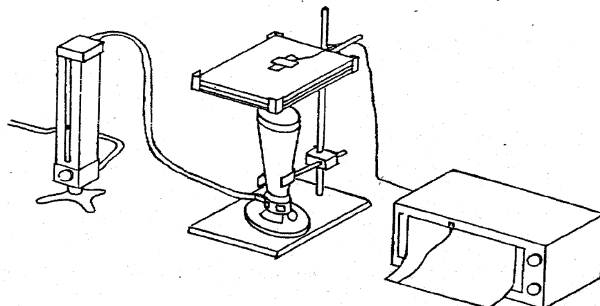
FIG. 1 Test Apparatus
