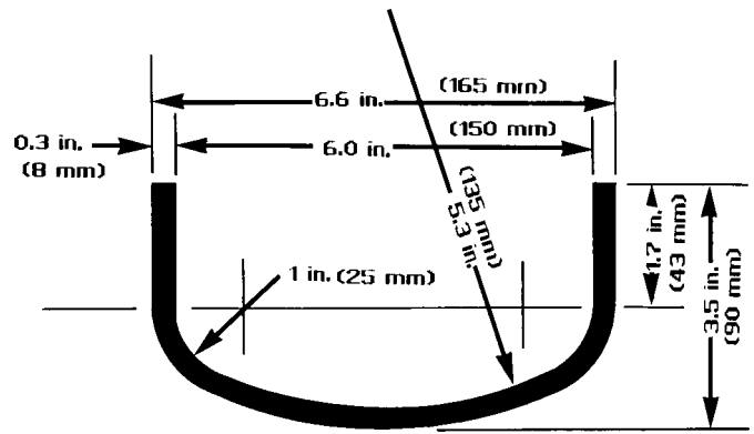
FIG. 12 Weld Cap
