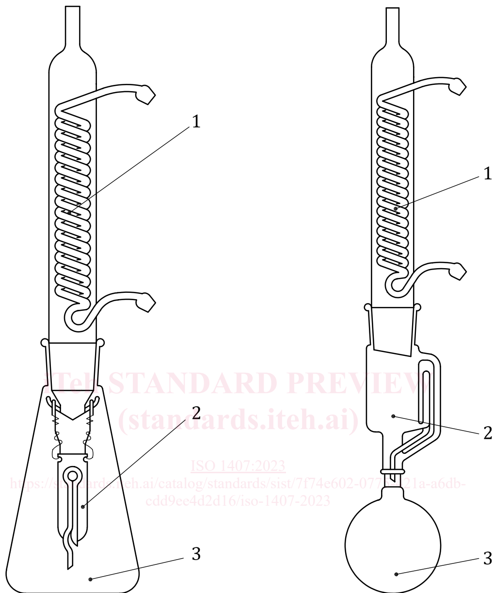
a) Appareil d'extraction entièrement en verre de type Kumagawa
