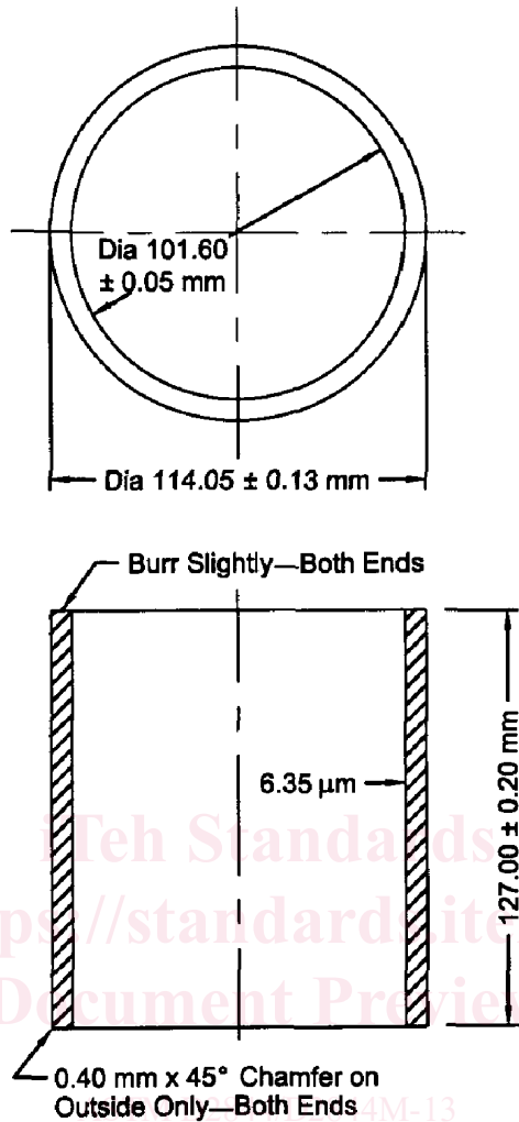
FIG. 3 Mold
