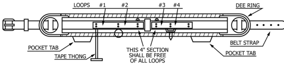
FIG. 13 Body Belt Nomenclature
