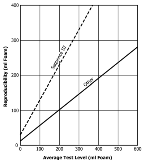
FIG. 4 Precision Chart—Reproducibility
