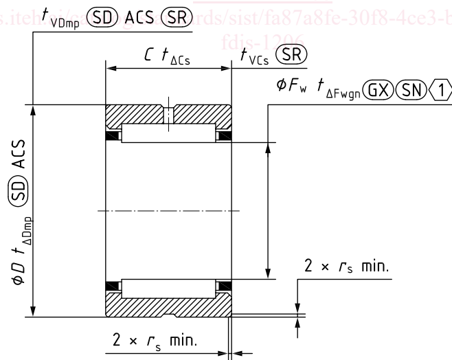
Figure 1 — Spécifications GPS des roulements à aiguilles avec bague intérieure
