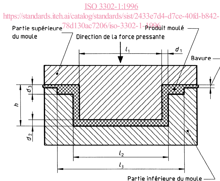
Figure 1 — Moule de compression et produit moulé (représentation schématique)
