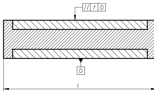
Figure 2 — Exemple de tolérance de parallélisme: structure en sandwich
