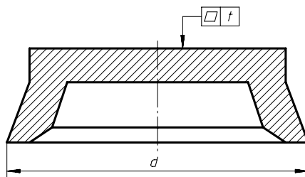
Figure 1 — Exemple de tolérance de planéité
