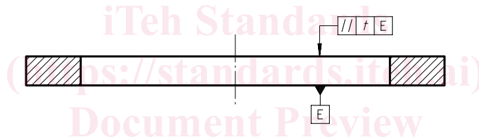
Figure 3 — Exemple de tolérance de parallélisme: section coupée de produit extrudé
