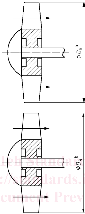
Figure 1 — Impeller — Centrifugal fan
