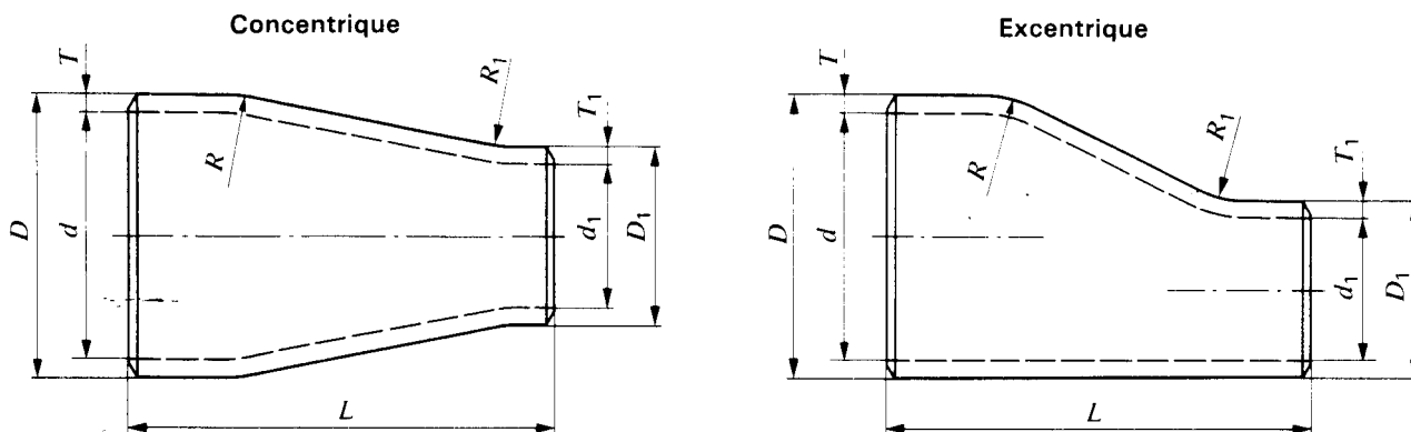
Figure 3 – Réductions concentriques et excentriques
