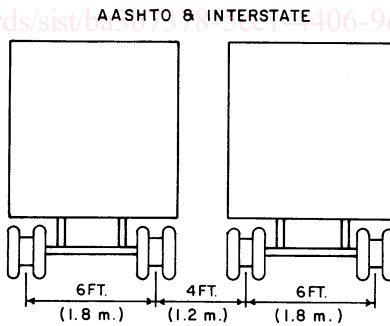
FIG. 1 Live Load Spacing
