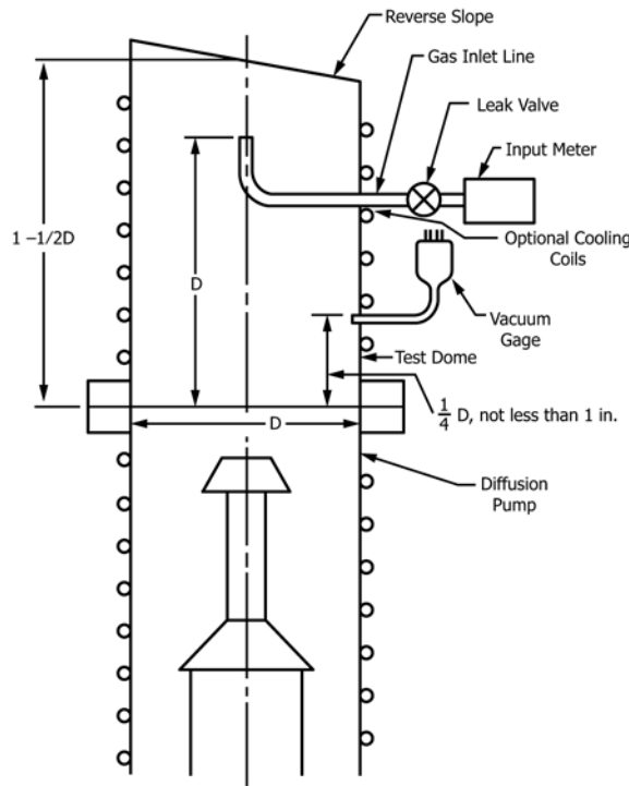
FIG. 1 Test Dome Dimensions
