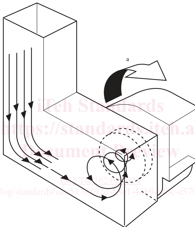
Figure 1 — Profils de vitesses non-uniformes au refoulement d'un ventilateur
