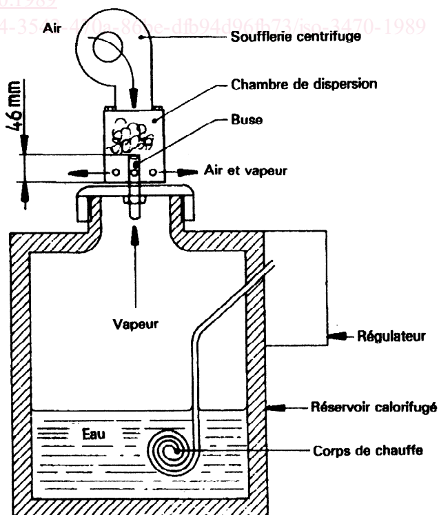
Figure 1 — Générateur de vapeur type
