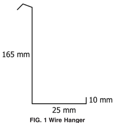
FIG. 1 Wire Hanger
