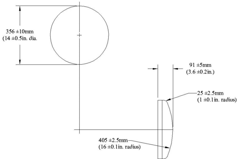
FIG. 4 Impact Platen
