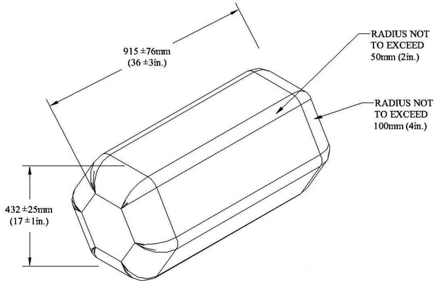
FIG. 3 Roller
