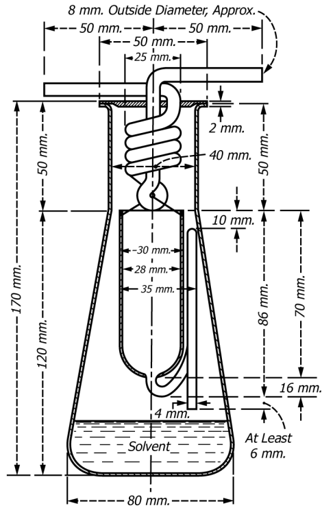
FIG. 1 Extraction Apparatus
