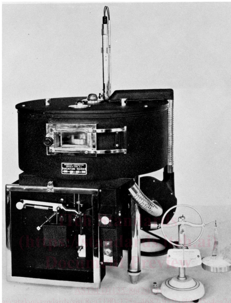
FIG. 1 Brabender Moisture Tester
