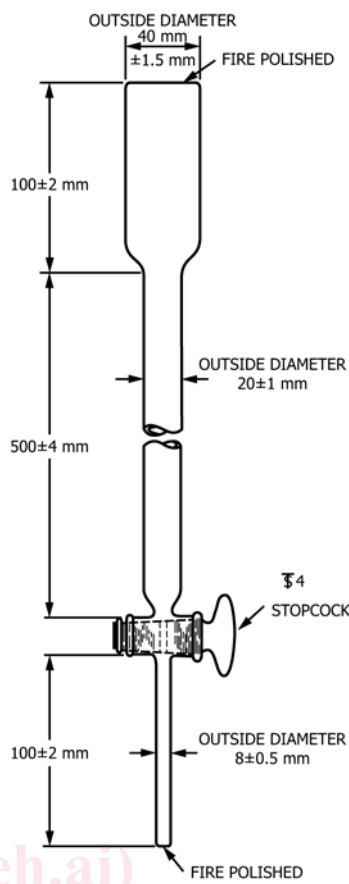
FIG. 1 Jones Reductor
