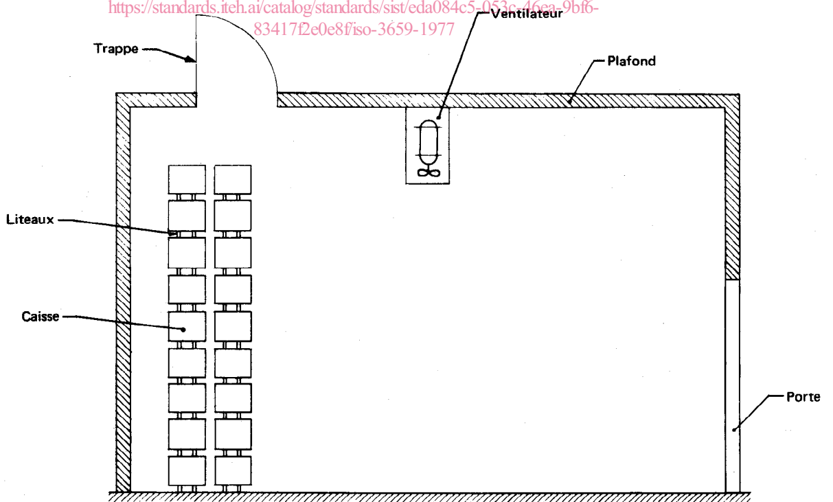
FIGURE 2 - Schéma d'une chambre de maturation de type rudimentaire
