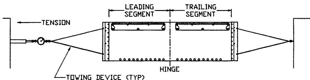
FIG. 1 Test Bed
