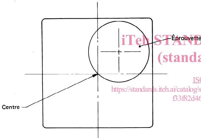
FIGURE — Prélèvement d'une éprouvette
