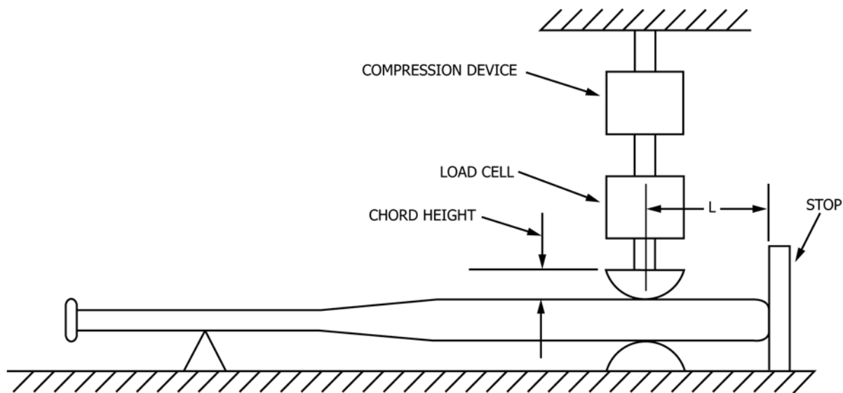
FIG. 1 Test Apparatus
